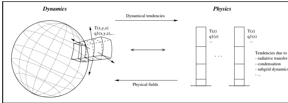
FIG. 2.1 – Interface physique/dynamique
