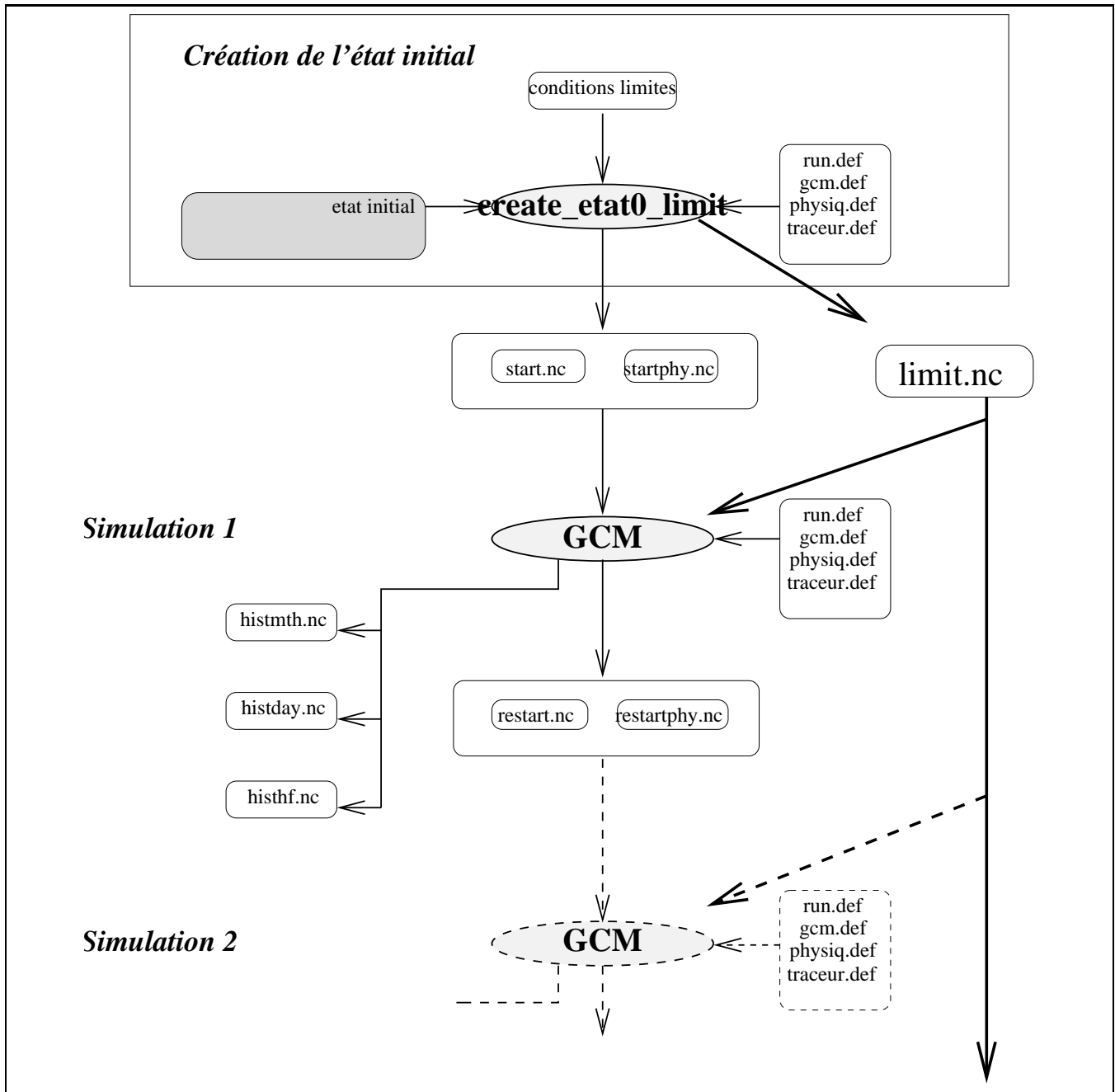
FIG. 6.4 – Entrées/Sorties
