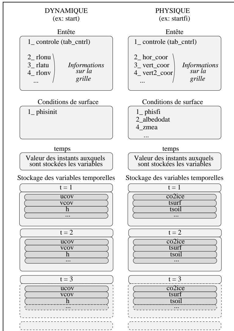
FIG. 6.3 – Organisation des fichiers NetCDF
