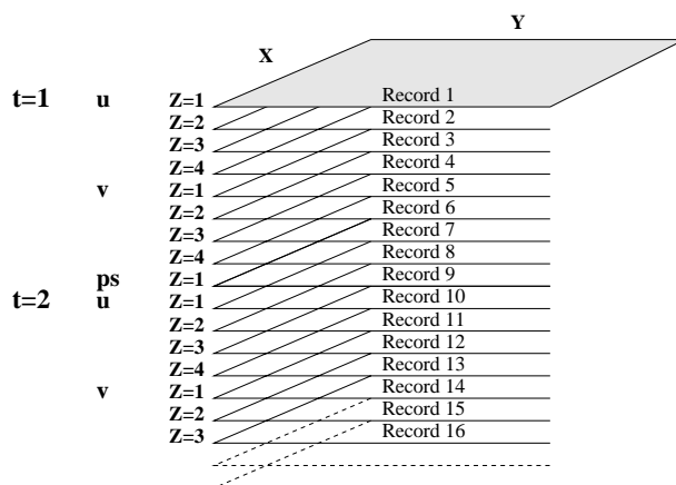
FIG. 6.2 – Exemple de stockage des vents u et v (champs 4D : X,Y,Z et t), et de la pression de surface ps (champ 3D : X,Y et t)
