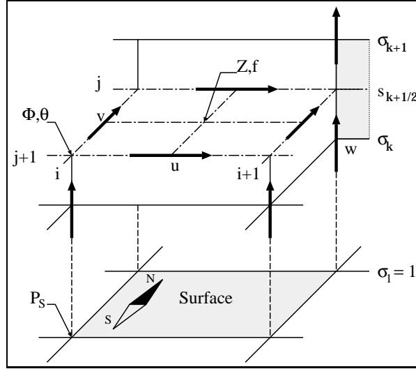
FIG. 3.2 – Disposition des variables dans la grille du LMD
