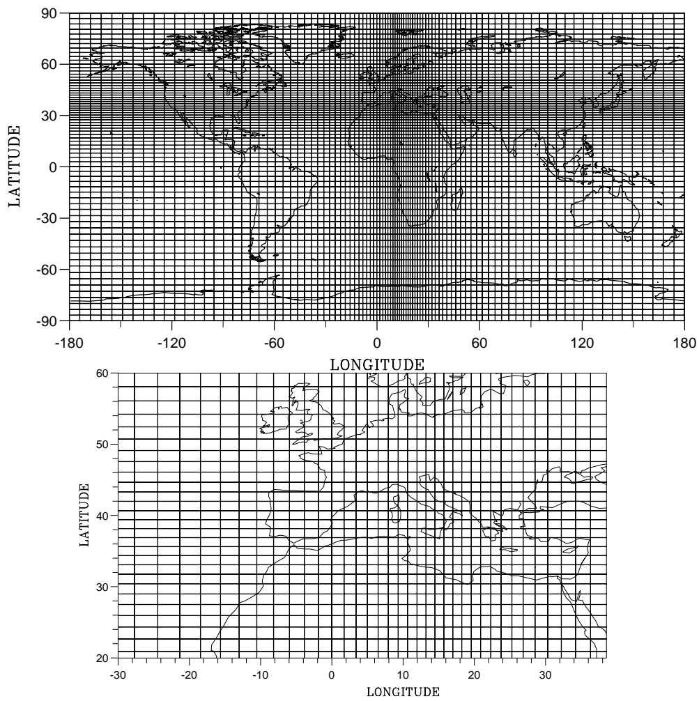
FIG. 3.1 – Grille obtenue avec 96 points en longitude et 73 en latitude et un zoom d'un facteur 3 centré sur la méditerranée (grille utilisée au laboratoire par Ali Harzallah)
