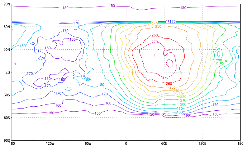
FIG. 6.1 – Exemple de visualisation sous GrADS des données de température à un instant donné
